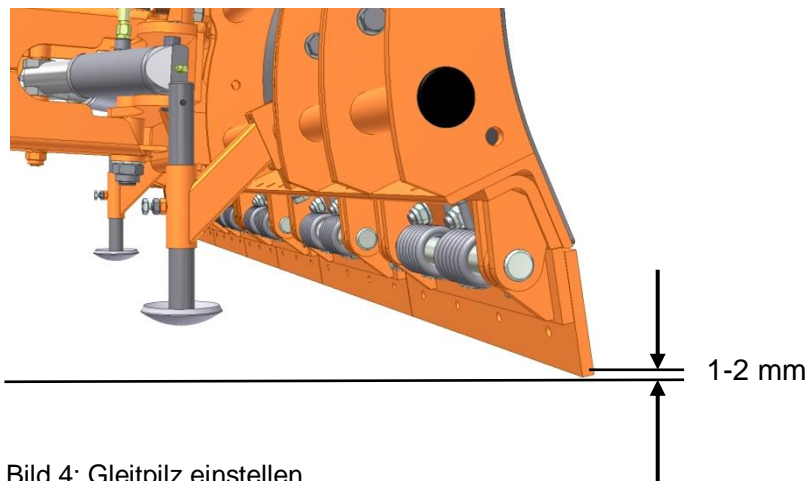
Bild 4: Gleitpilz einstellen
