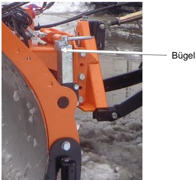
Bild 6: Teleskopfuß sichern
