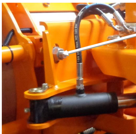
Bild 8: Einstellen des Auflegewinkels - Stellschraube
